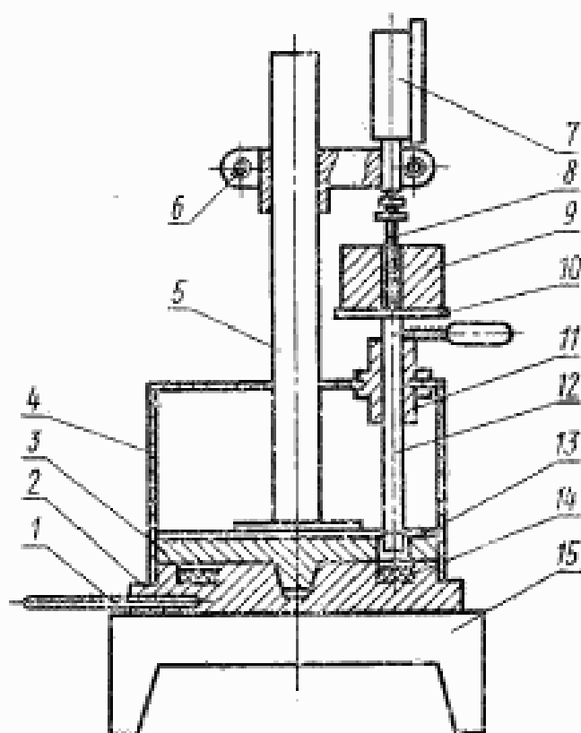
1—термометр; 2—нижняя плита; 3—верхняя плита; 4—кожух; 5—стойка; 6—держатель индикаторов; 7—индикатор; 8—узел индикатора; 9—груз; 10—площадка груза; 11—направляющая втулка; 12—штока; 13—пуансон; 14—образец; 15—нагреватель.
